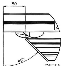
DETTAGLIO C SCALA 1:2
