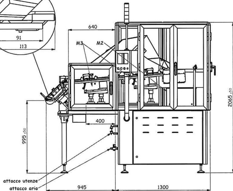
DETTAGLIO A SCALA 1 : 2
